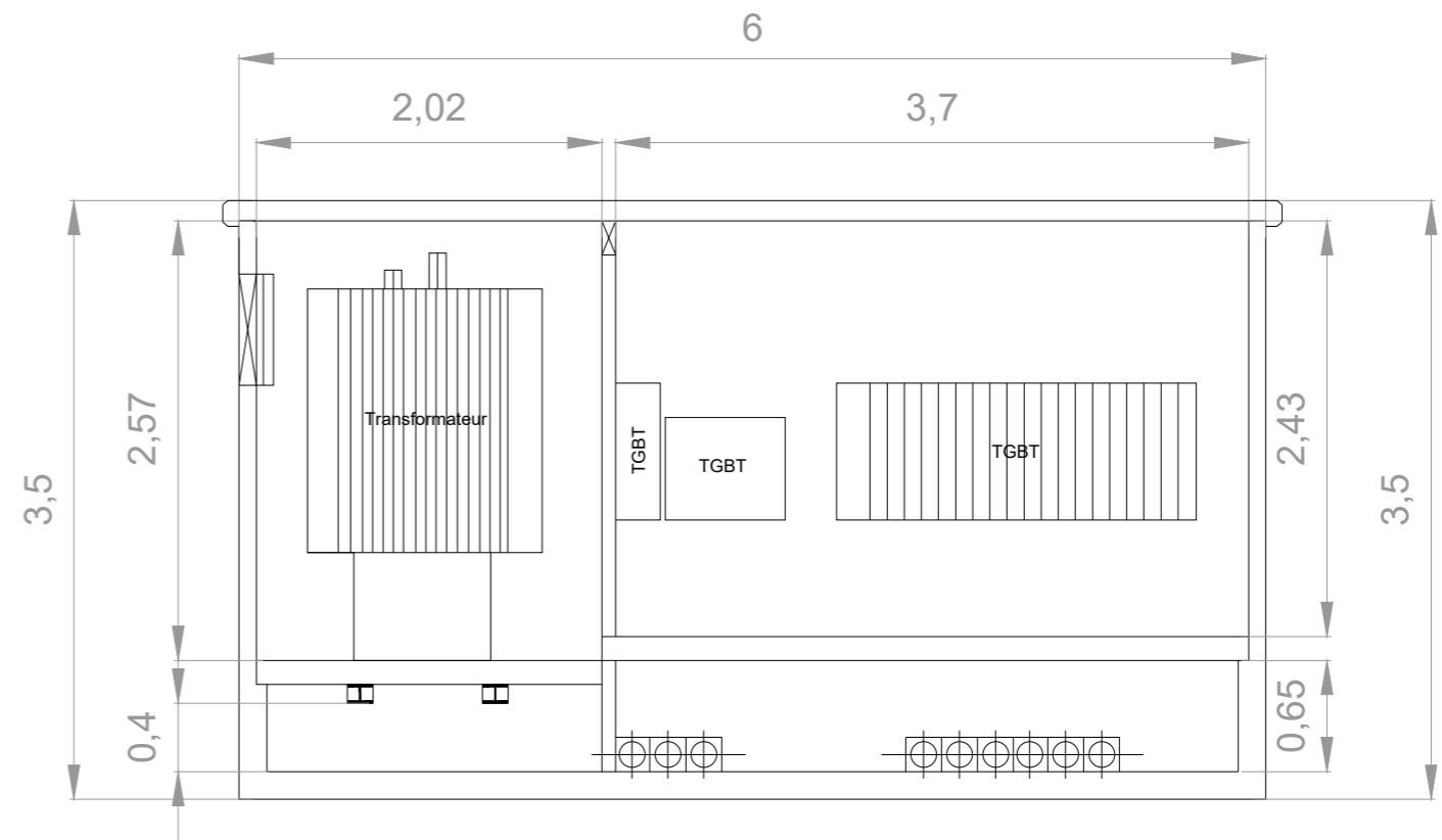
Coupe A-A'
