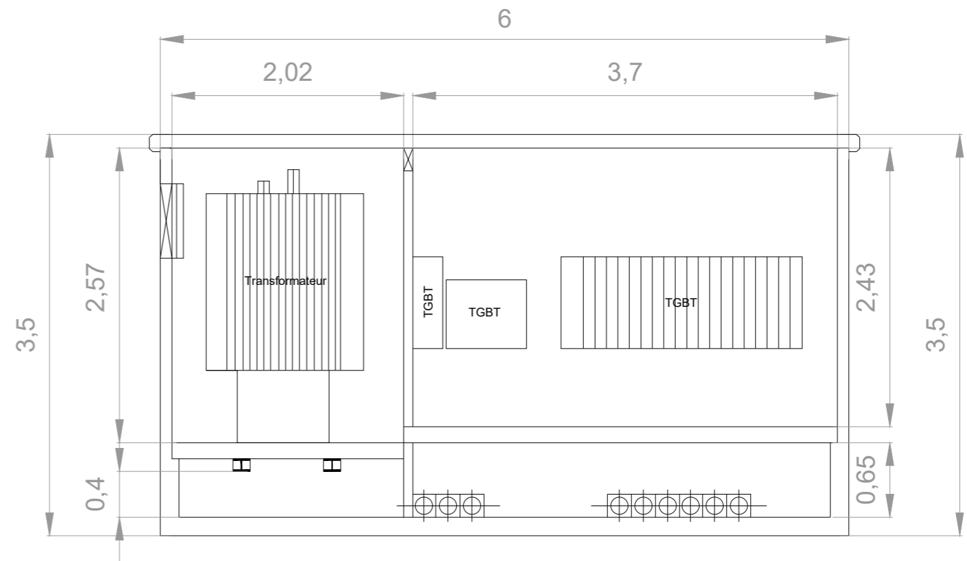
Coupe A-A'
